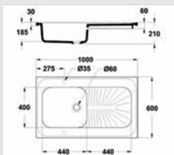
EVIL 4560 Evier 1 Cuve - 1 Egouttoir
