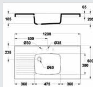
EVIL 3663 Evier 1 Cuve - 2 Egouttoirs
